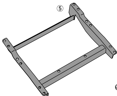
アダプター (RO、YO) ×1
