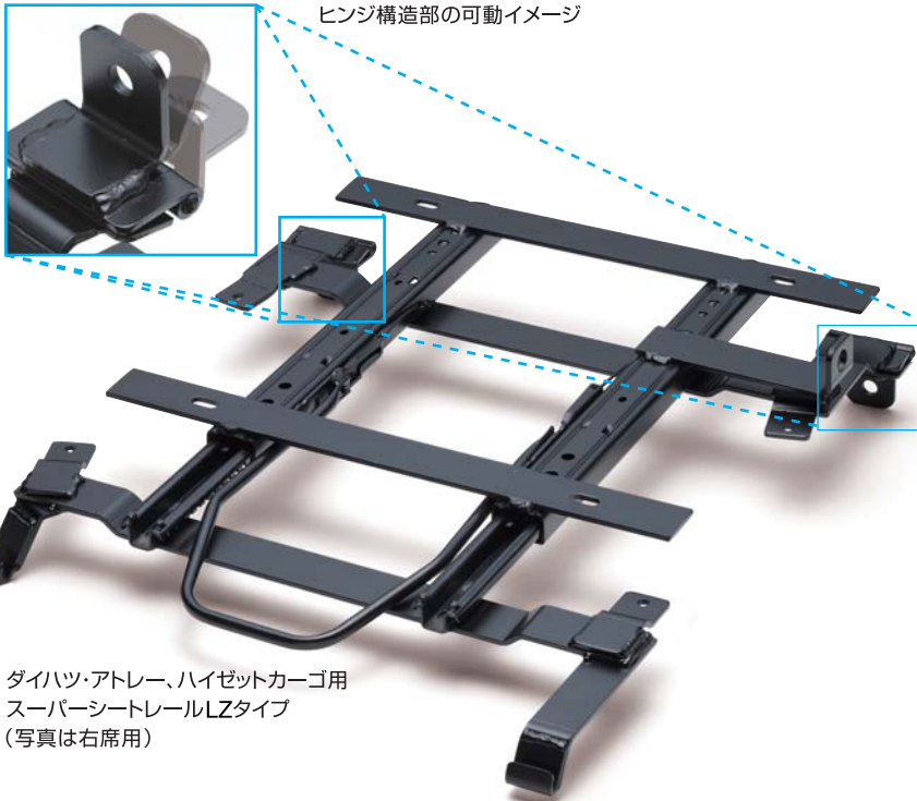
ヒンジ構造部の可動イメージ
